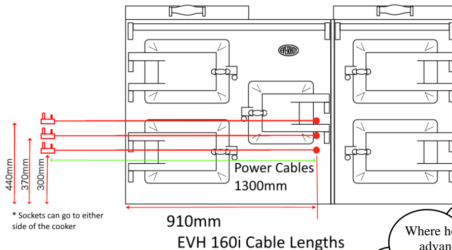
EVH160i dimensions
